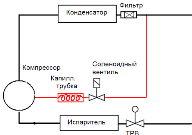
Рис 7: Впрыск жидкости
