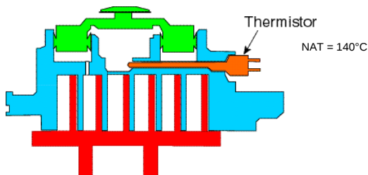
Рис 17: Расположение встроенного датчика температуры нагнетания
