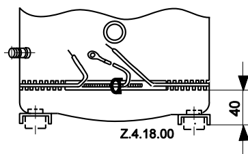
Рис 15: Положение подогревателя картера
