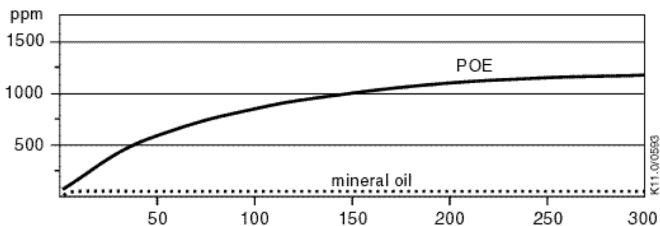
Рис 19: Сравнение уровней поглощения влаги ПЭМ и минеральным маслом по весу [ppm] при 25°C и 50% относительной влажности, h = час
