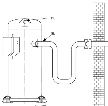
Рис 10: Конструкция всасывающего трубопровода
